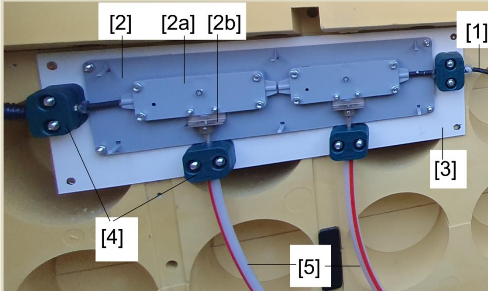
Einbruch-Meldesensor
